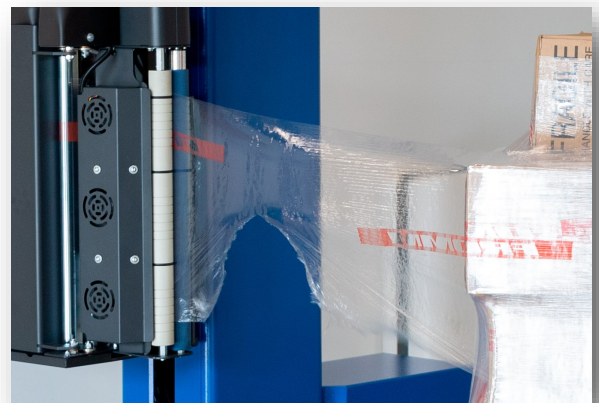
Abschneiden der Folie am Ende des Wickelzyklus
